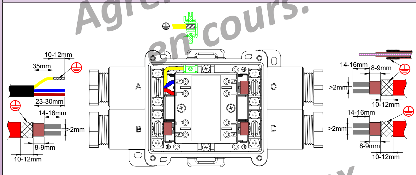
Modèle à 3 câbles chauffants et un câble d'alimentation
